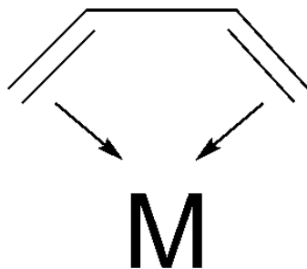
ジエン錯体
